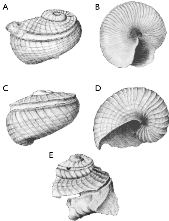
Fig. 8. Scissurella ( s. l. ) aliceae Schnetler, Lozouet & Pacaud 2001. A , B : MGUH 25759 (ex Rkz 119), width 1.9 mm, height 1.6 mm. C , D : MGUH 25758 (ex Rkz 120), width 1.8 mm. E : MGUH 30969 (ex Rkz 100), height 1.8 mm.
